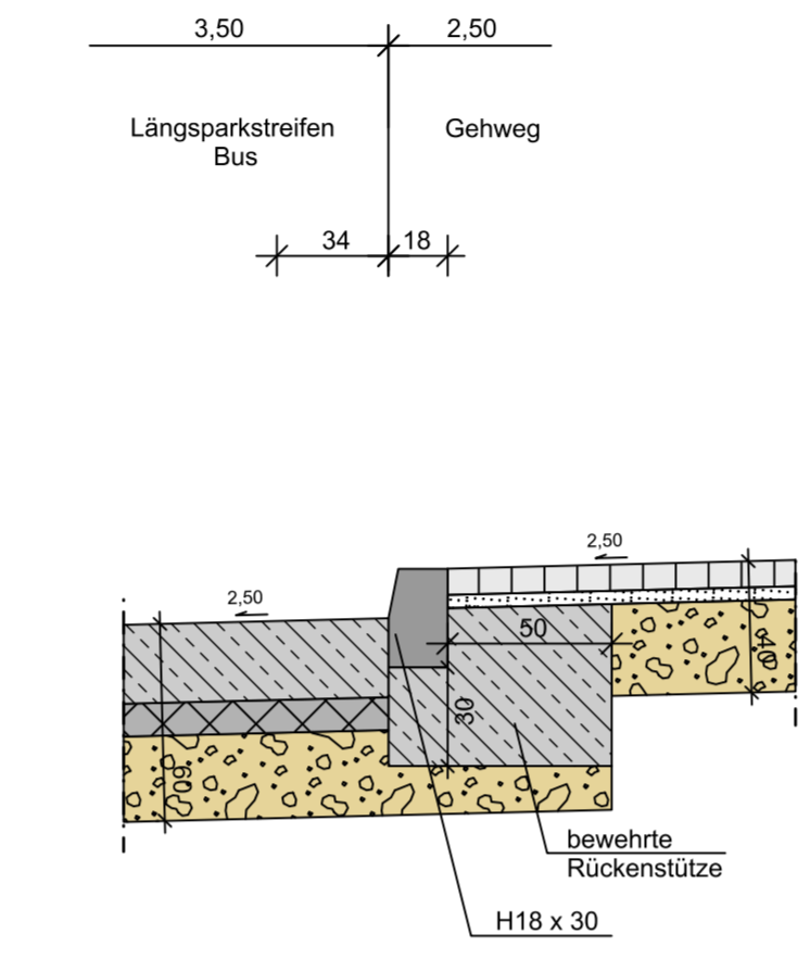
Detail F Maßstab 1 : 25
