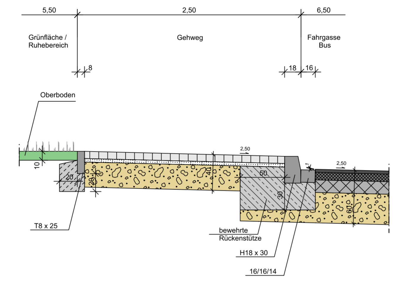
Detail C Maßstab 1 : 25
