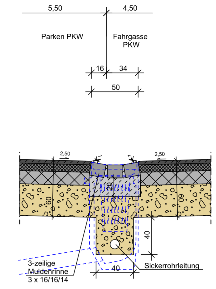
Detail G Maßstab 1 : 25
