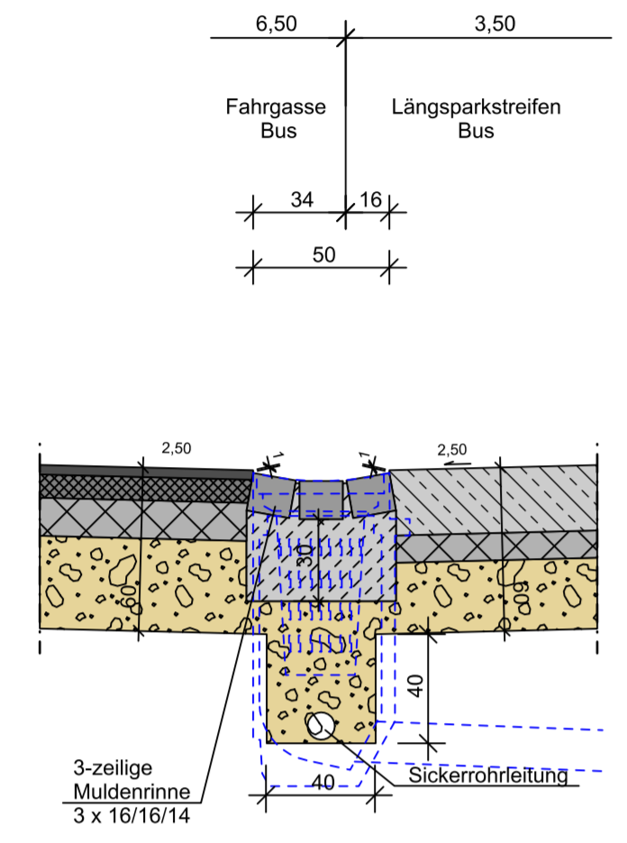
Detail A Maßstab 1 : 25
