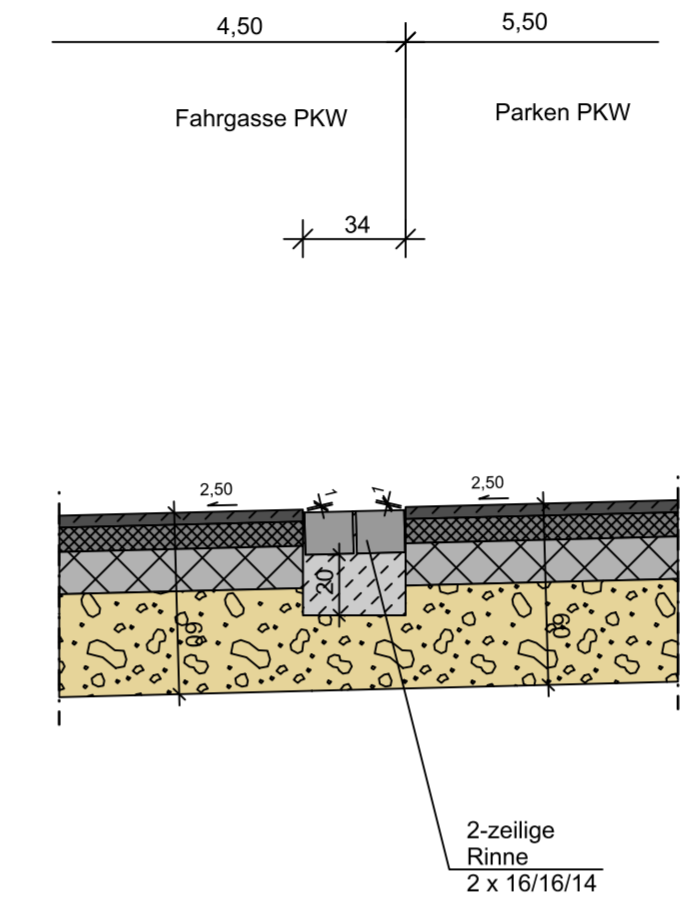
Detail H Maßstab 1 : 25
