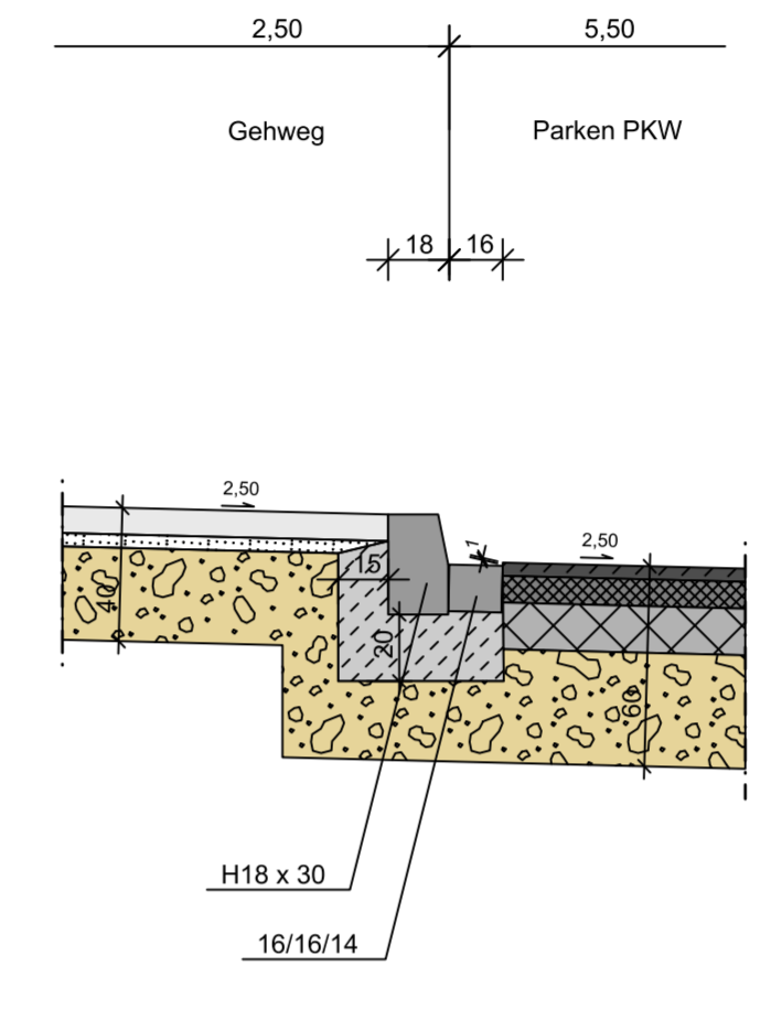
Detail I Maßstab 1 : 25
