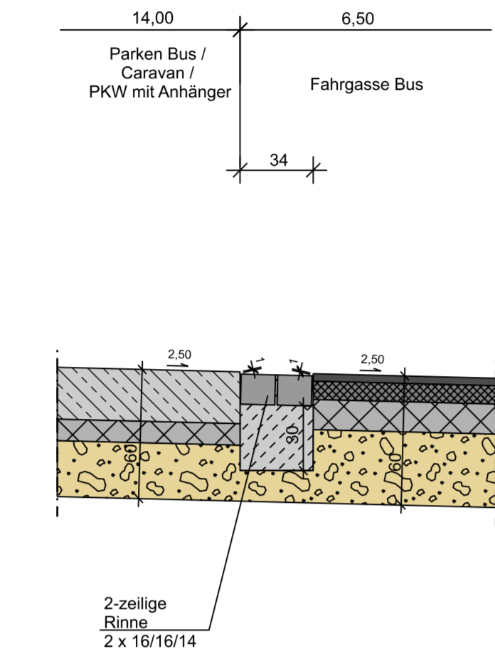
Detail B Maßstab 1 : 25
